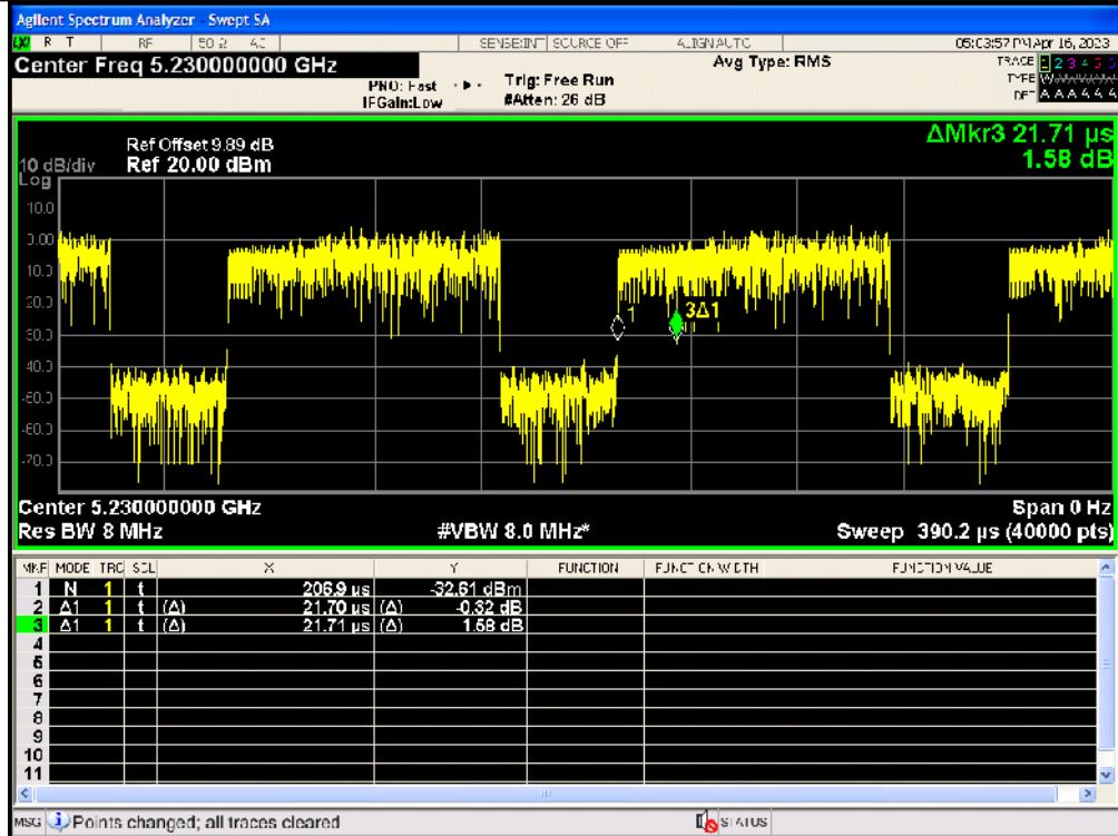
IEEE 802.11n_40MHz_Channel 46
