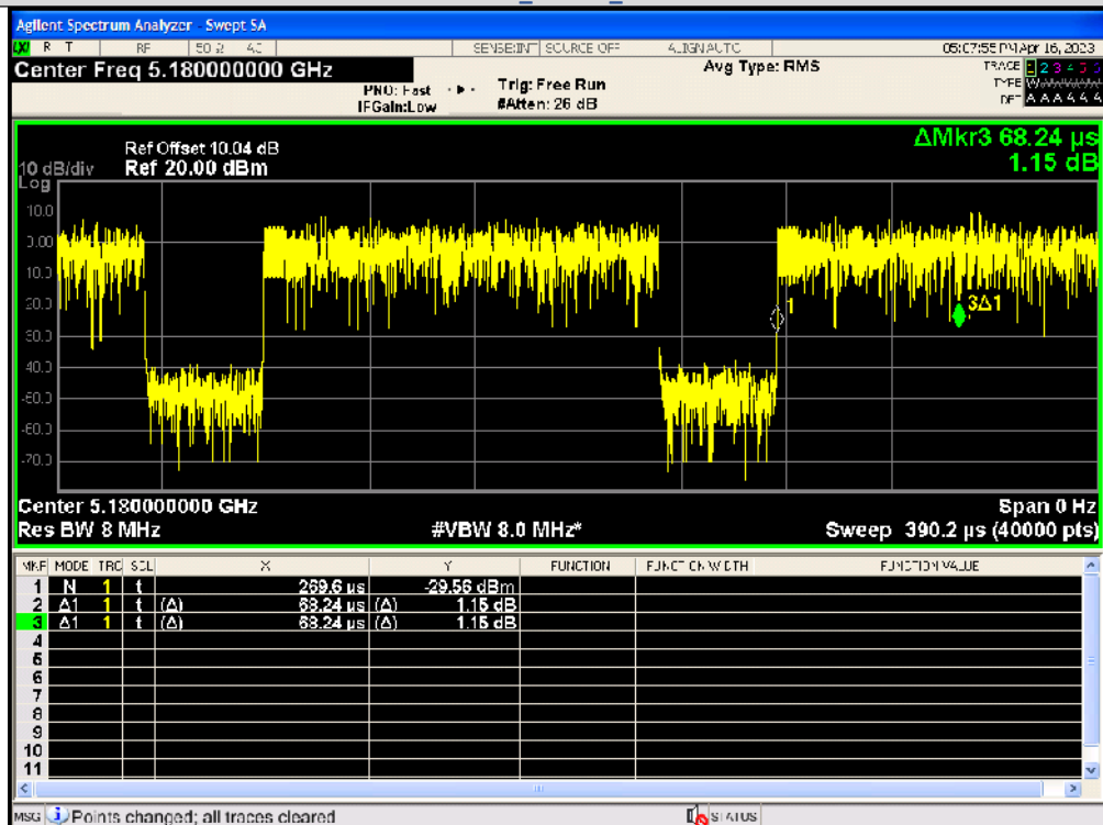
IEEE 802.11ac_20MHz_Channel 36
