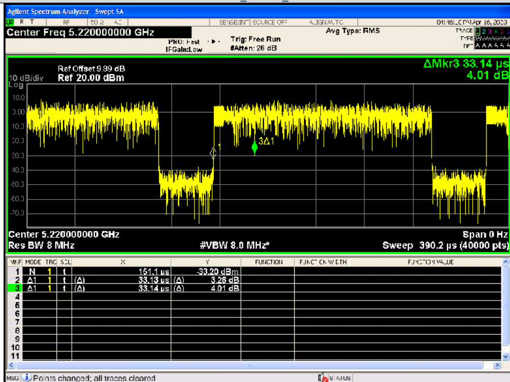
IEEE 802.11a_20MHz_Channel 44
