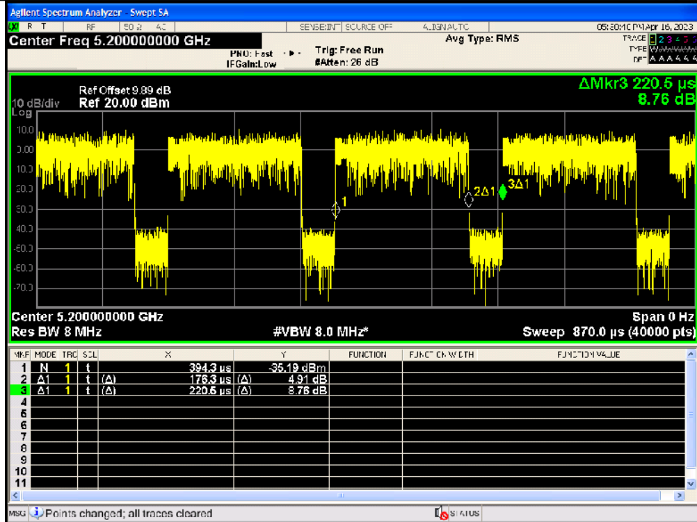
IEEE 802.11a_20MHz_Channel 40
