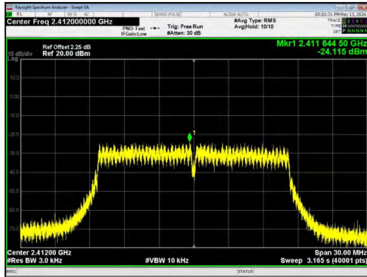
802.11g - CH01
