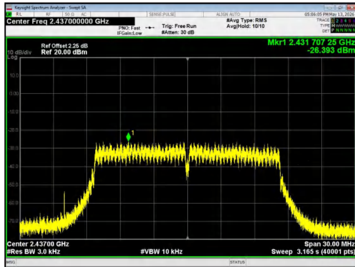
802.11g - CH06
