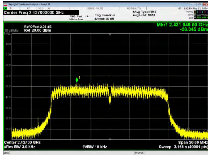
802.11n20 - CH06
