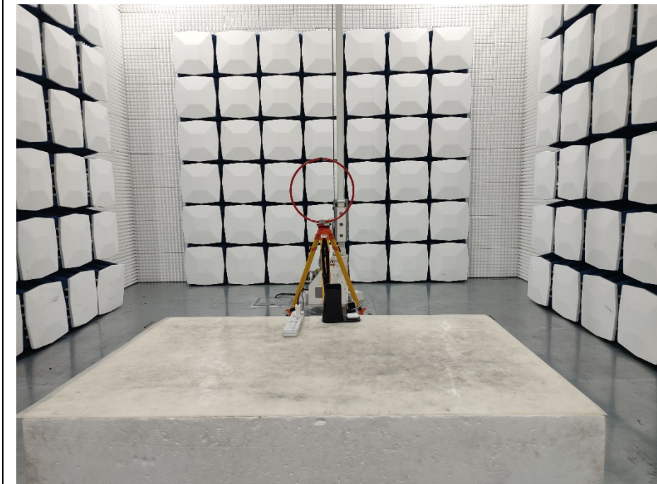
9KHz-30MHz
