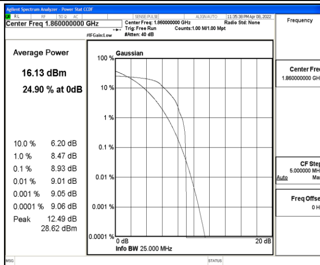
Band2-20MHz-QPSK-18700-1-0-Low-8.93-&lt;=13-PASS
