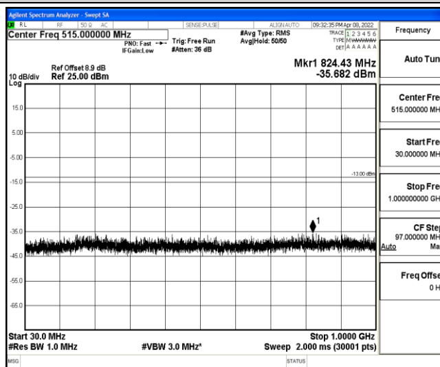
Band2-1.4MHz-QPSK-18900-1-0-Low-30-1000--35.68-PASS
