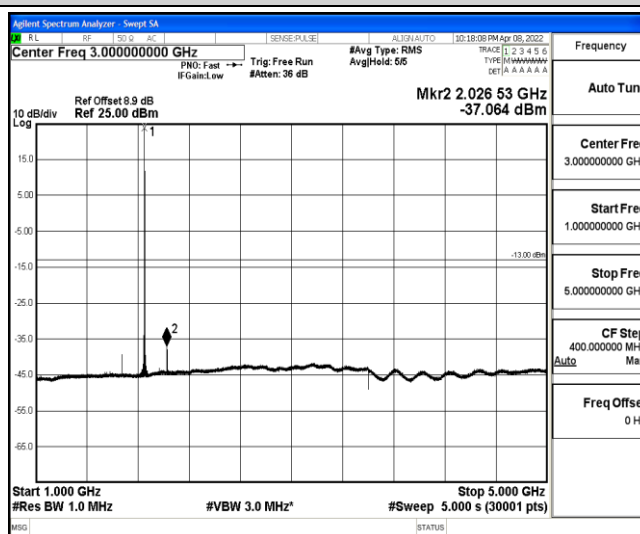
Band2-5MHz-QPSK-18625-1-0-Low-1000-5000--37.06-PASS
