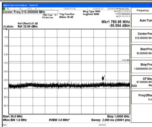
Band4-5MHz-QPSK-20175-1-0-Low-30-1000--35.55-PASS
