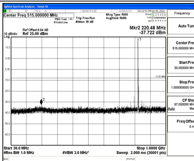
Band5-10MHz-QPSK-20450-1-0-Low-30-1000--37.72-PASS
