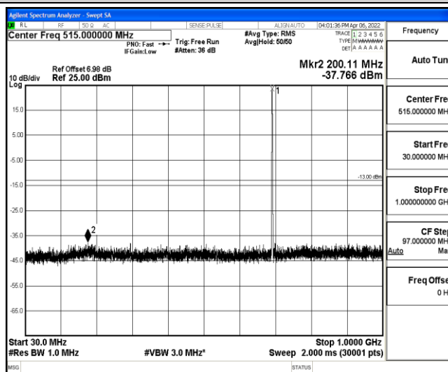
Band12-5MHz-QPSK-23035-1-0-Low-30-1000--37.77-PASS
