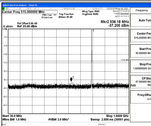
Band12-1.4MHz-16QAM-23017-1-0-Low-30-1000--37.21-PASS
