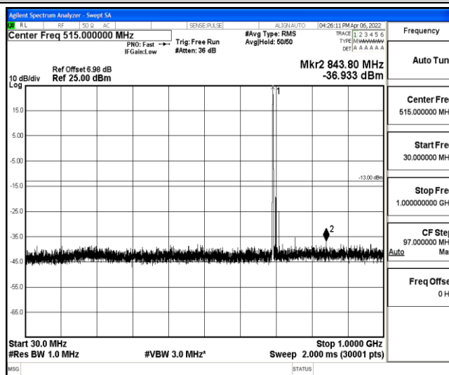
Band12-10MHz-QPSK-23060-1-0-Low-30-1000--36.93-PASS
