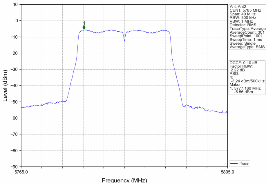
802.11n(HT20)_MCH_5785MHz_MIMO_NTNV
