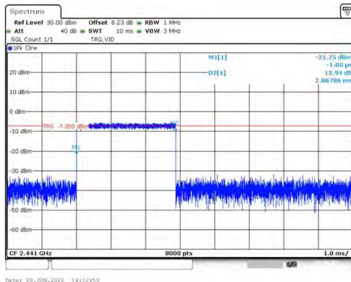
\pi/4 -DQPSK mode-2DH5
