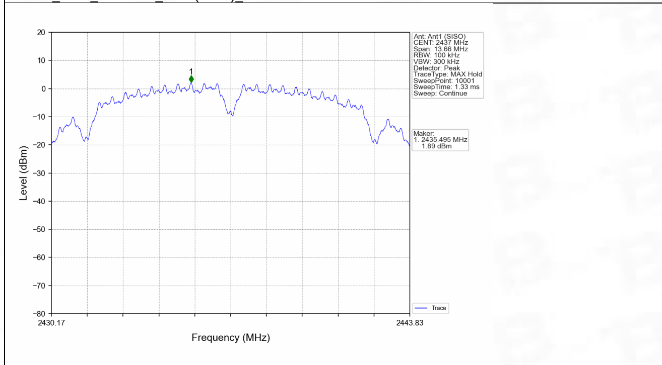
802.11b_MCH_2437MHz_Ant1 (SISO)_NTNV
