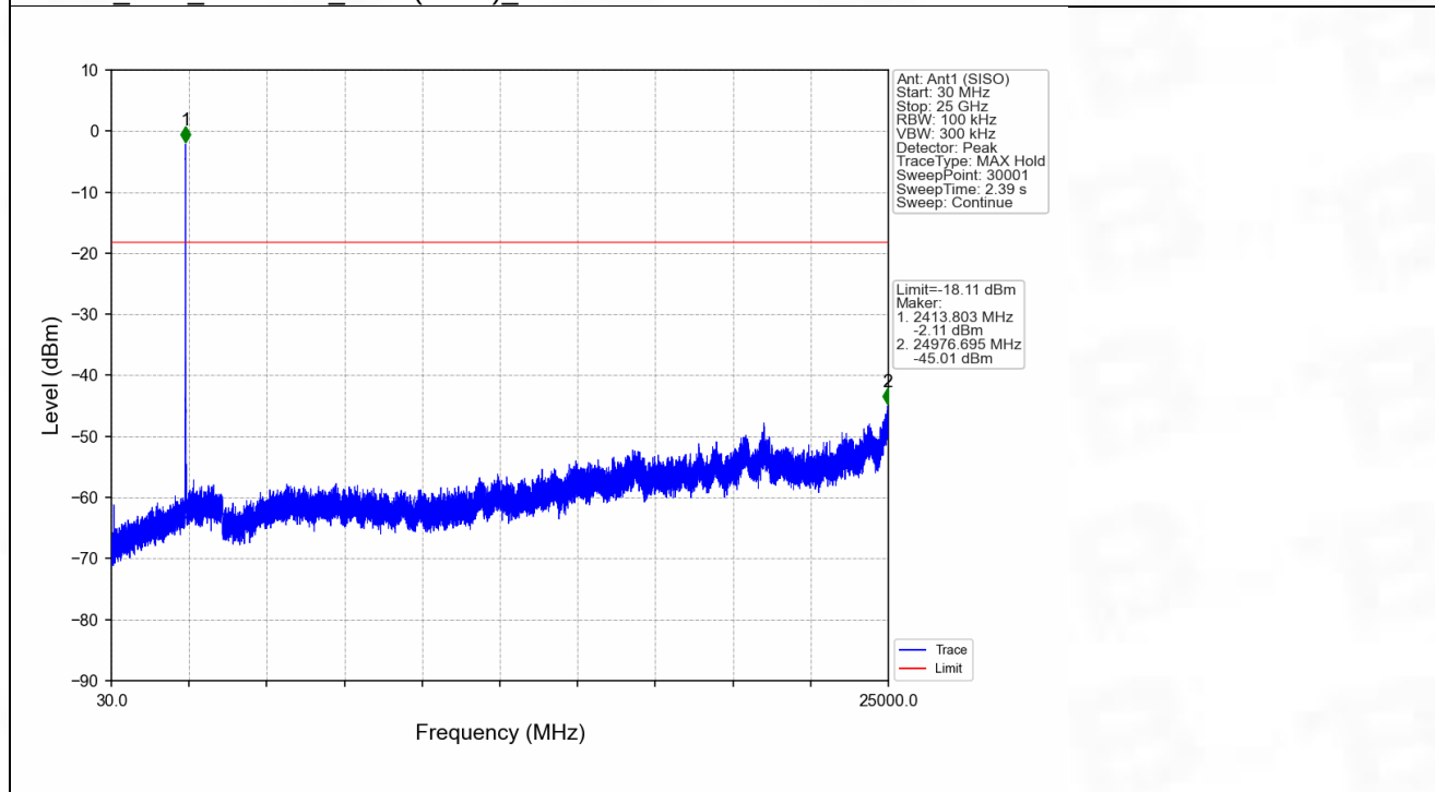
802.11b_LCH_2412MHz_Ant1 (SISO)_NTNV
