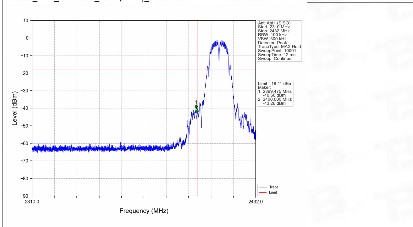
802.11b_LCH_2412MHz_Ant1 (SISO)_NTNV
