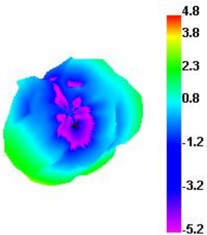
5850.000MHz E1
