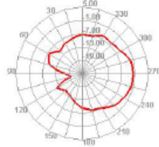
5150.000MHz H
