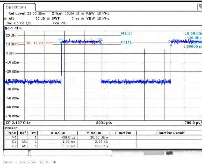
11G-CDD_Ant2_2437
