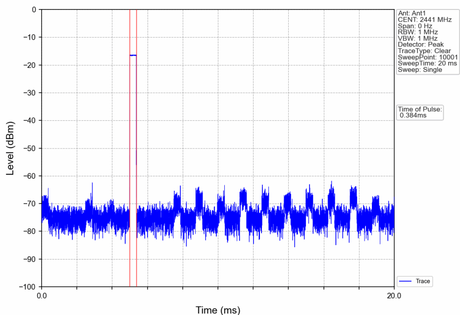
GFSK_DH1_HOPP_Ant1_NTNV
