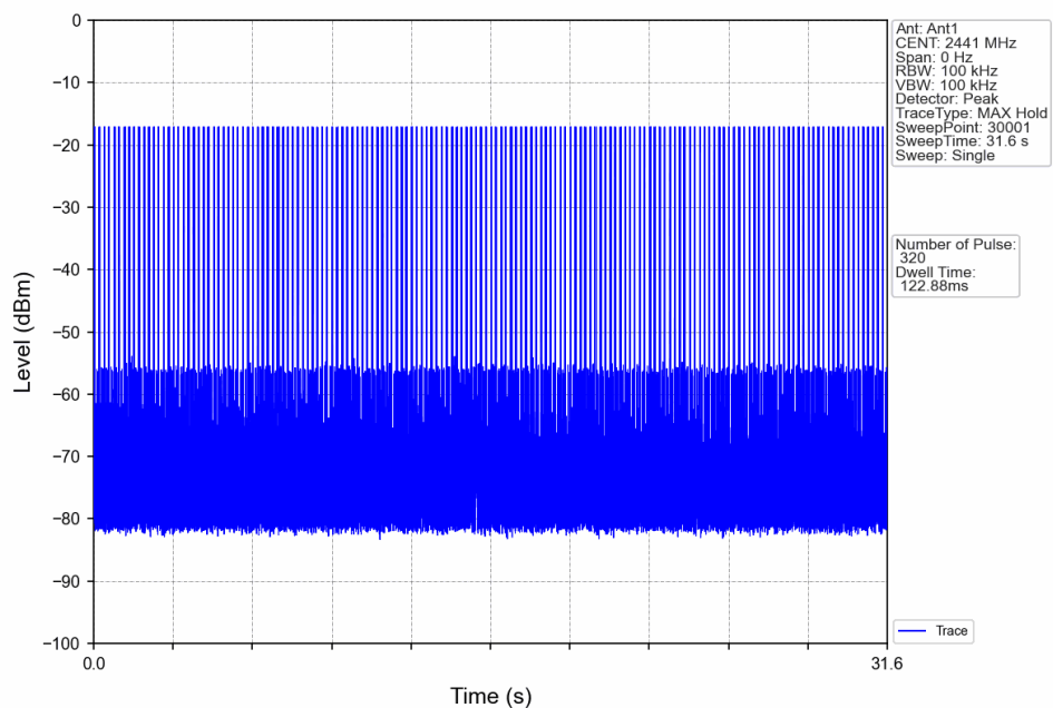
GFSK_DH1_HOPP_Ant1_NTNV
