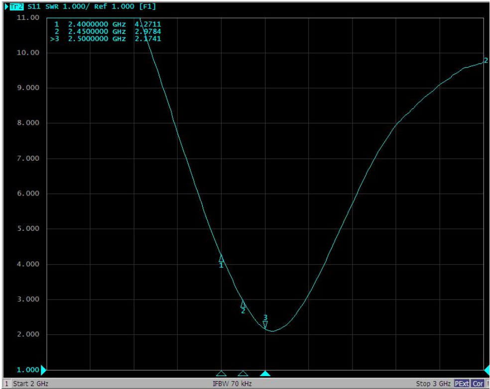
V.S.W.R
