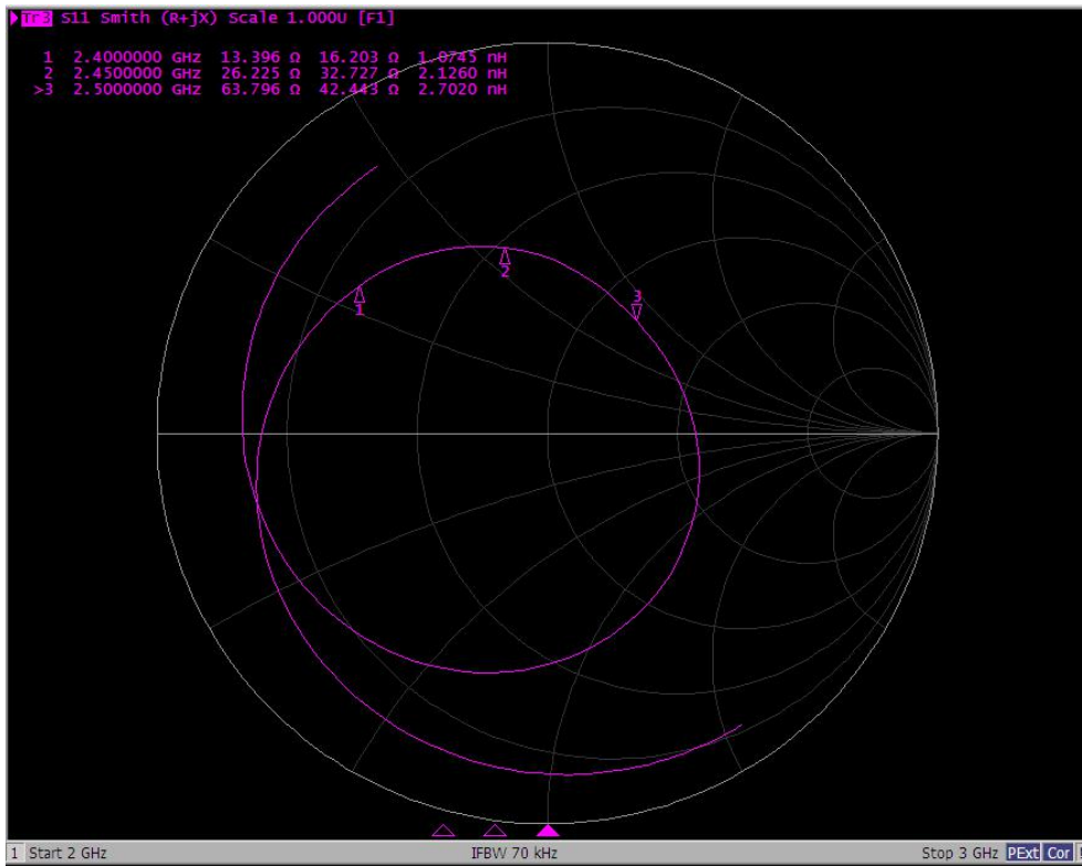
Smith Chat
