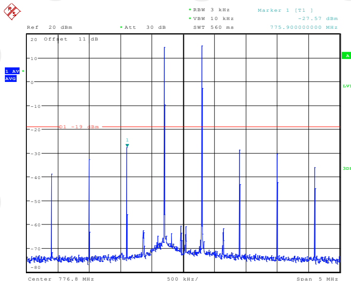
Upper700MHz Pre AGC, UL
