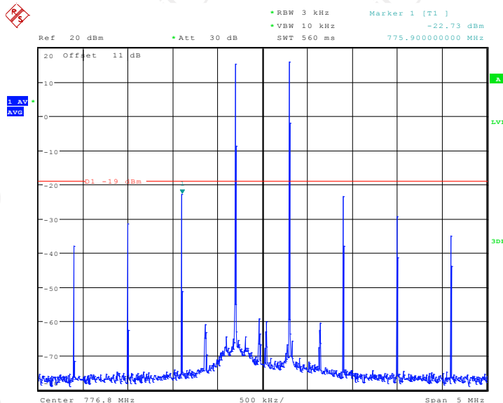
Upper700MHz AGC +10dB , UL
