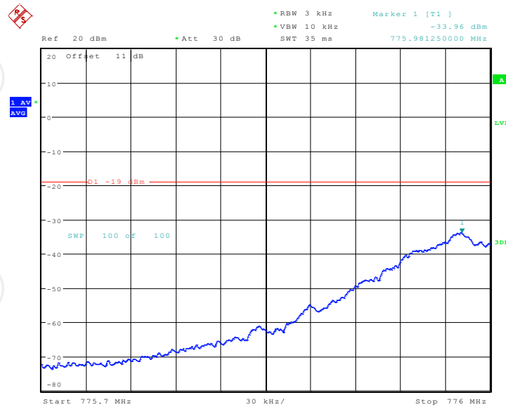
Upper700MHz GSM UL Left Side Pre AGC
