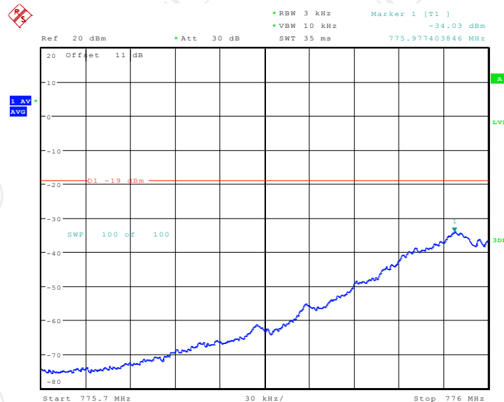
Upper700MHz GSM UL Left Side Pre AGC+10dB
