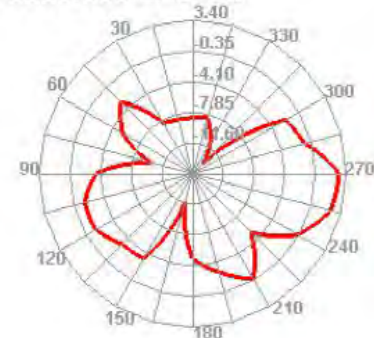
5850.000MHz E2
