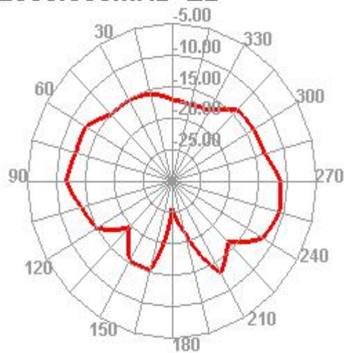
2500.000MHz E2
