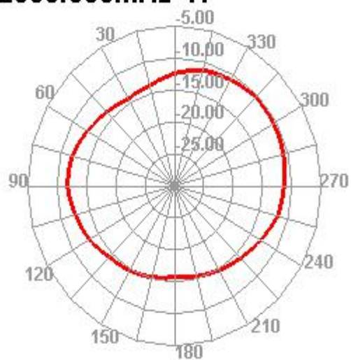
2500.000MHz H
