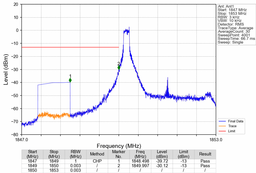
Band2_3MHz_QPSK_LCH_1851.5MHz_RB_1_0_NTNV
