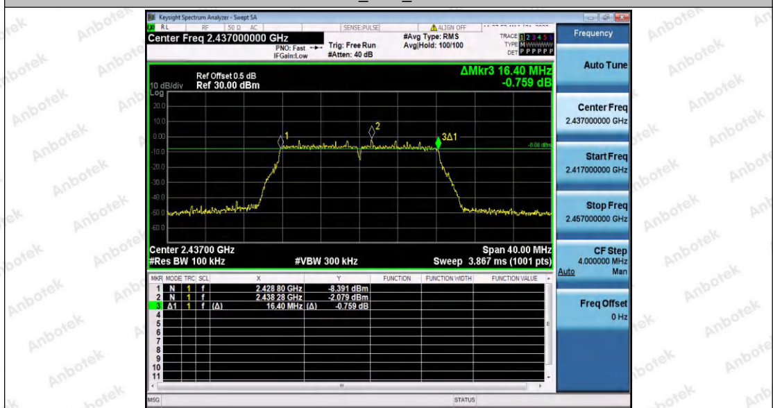
11G_Ant1_2437
