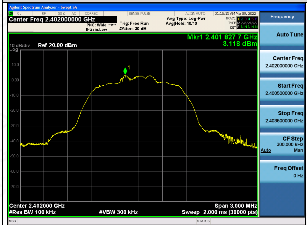
Test_Graph_EDR_ANT1_2402_2Mbps_Reference Level
