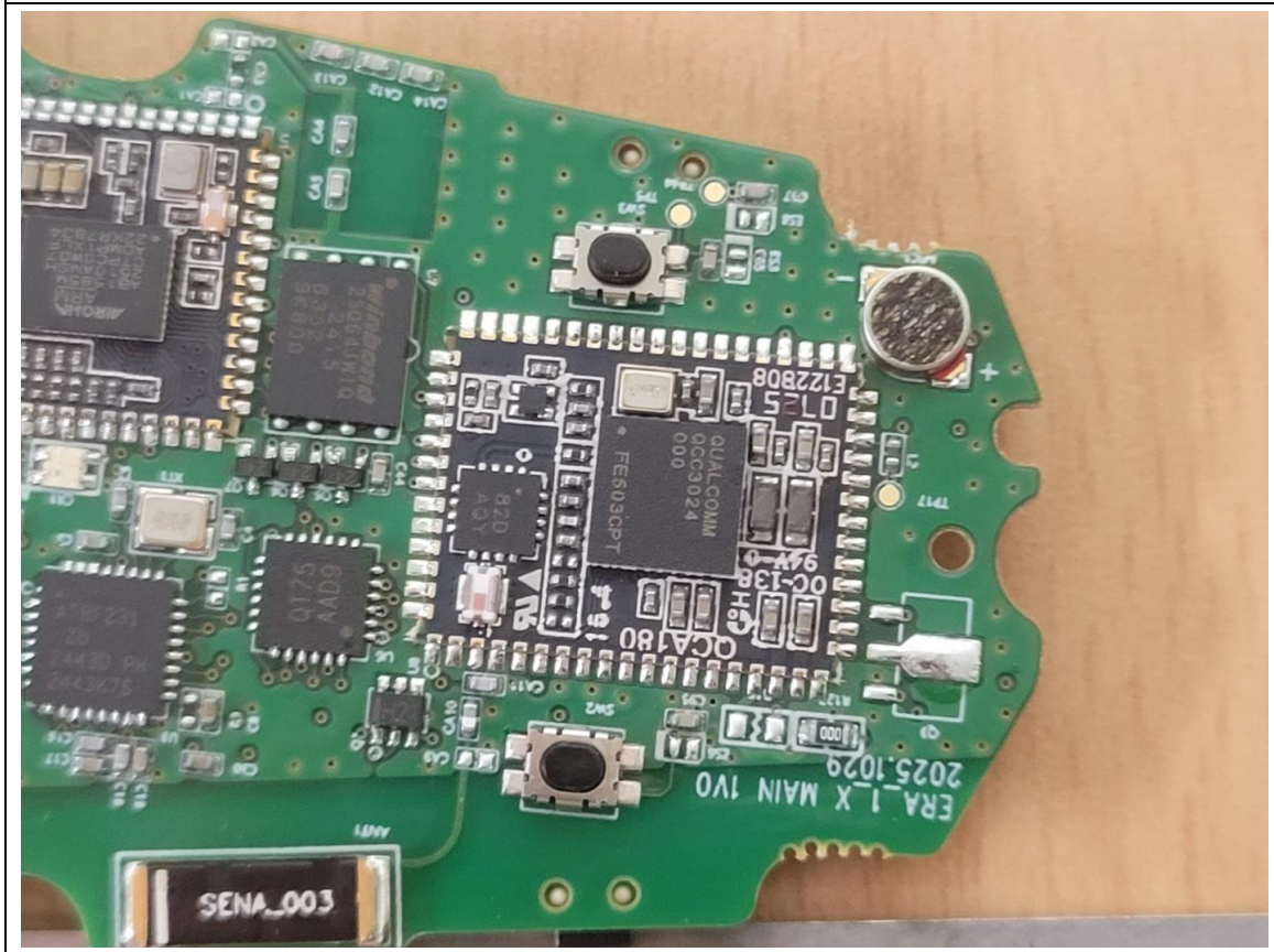
BT1 Module
