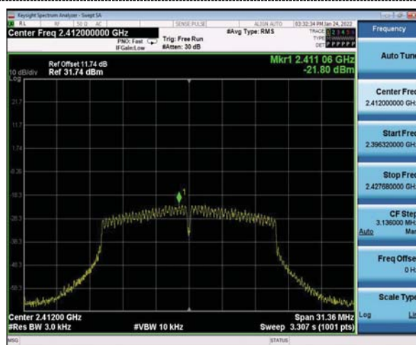
CH01
