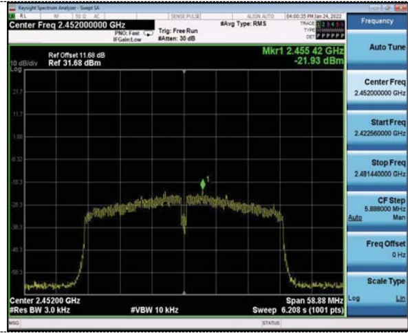
CH09
