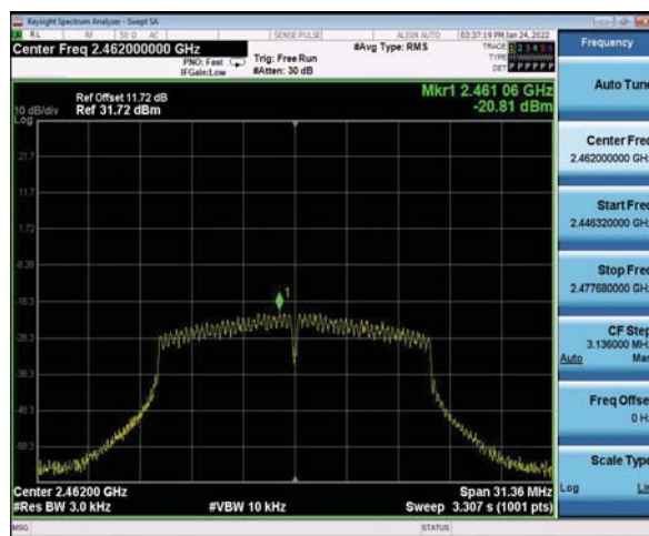
CH11
