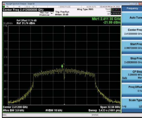
CH01
