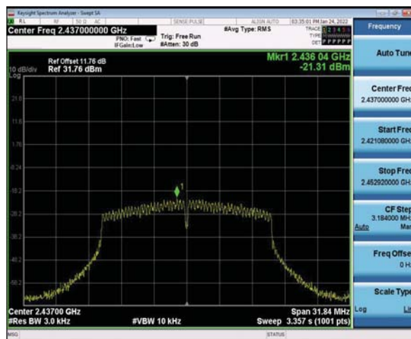
CH06
