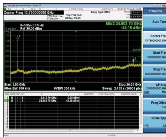
1GHz -26.5GHz
