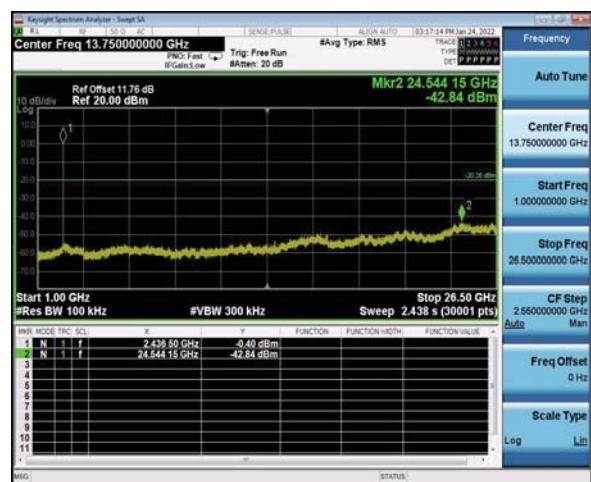
1GHz -26.5GHz
