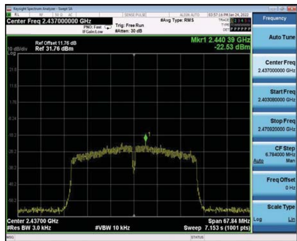
CH06
