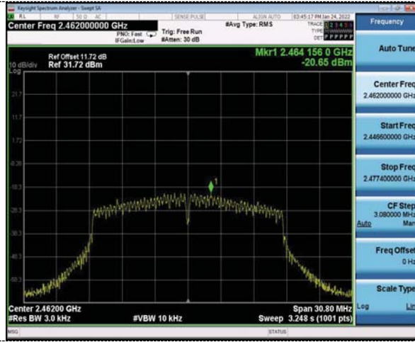
CH11
