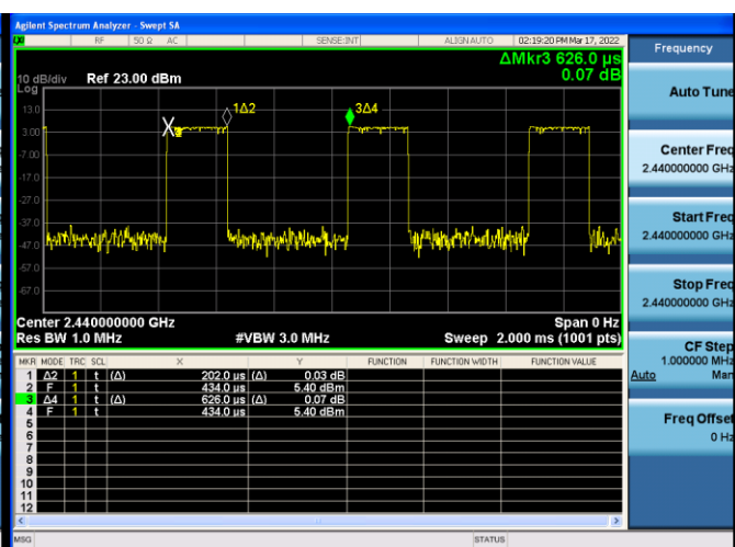
Mode 4 CH19 2440MHz
