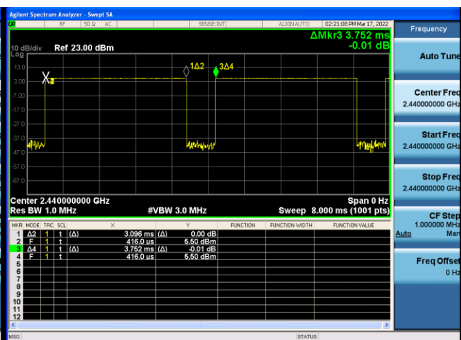
Mode 4 CH19 2440MHz
