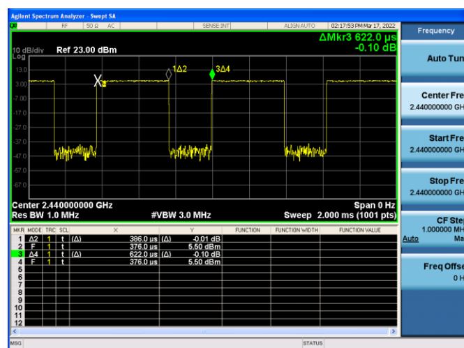
Mode 3 CH19 2440MHz
