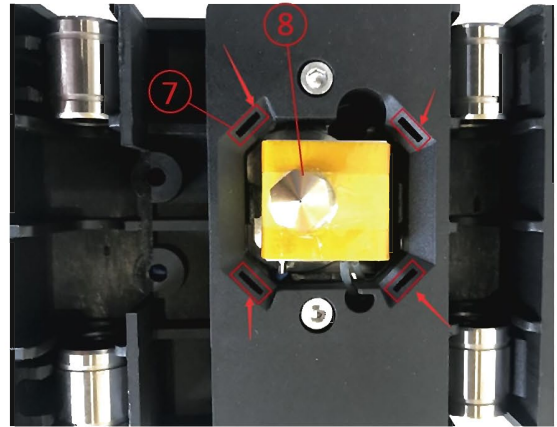
Extruder
