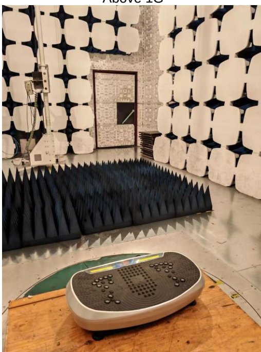
Above 1G
