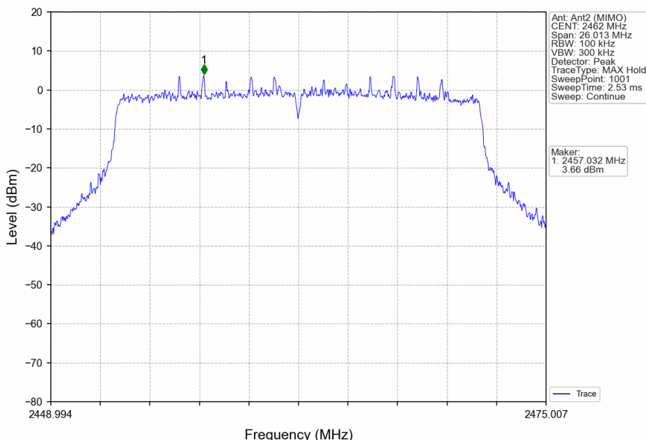
802.11ax(HEW20)_HCH_2462MHz_RU242_Left_Ant2 (MIMO)_NTNV
