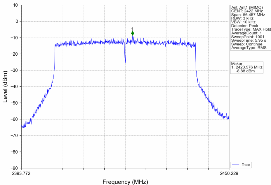
802.11ax(HEW40)_LCH_2422MHz_RU484_Left_Ant1 (MIMO)_NTNV
