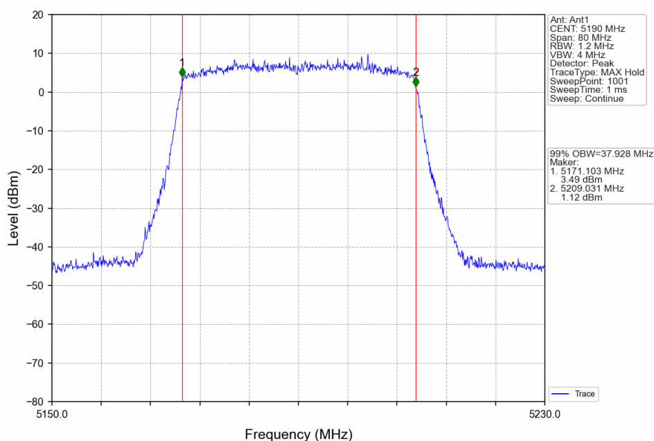
802.11ax(HEW40)_LCH_5190MHz_RU484_Left_Ant1_NTNV
