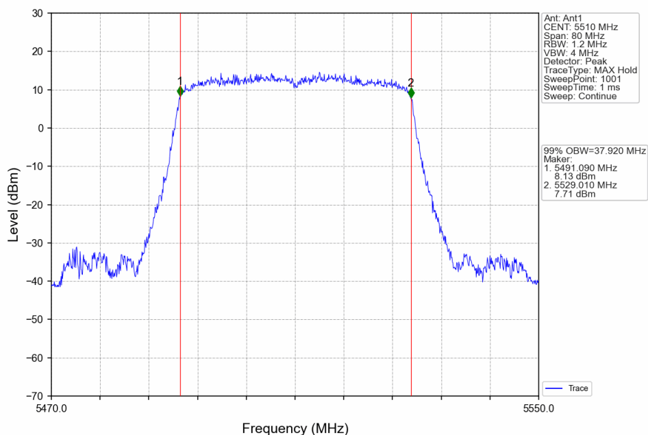
802.11ax(HEW40)_LCH_5510MHz_RU484_Left_Ant1_NTNV
