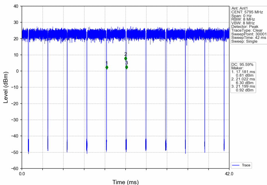
802.11ax(HEW40)_HCH_5795MHz_RU484_Left_Ant1_NTNV
