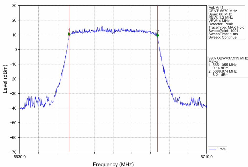
802.11ax(HEW40)_HCH_5670MHz_RU484_Left_Ant1_NTNV
