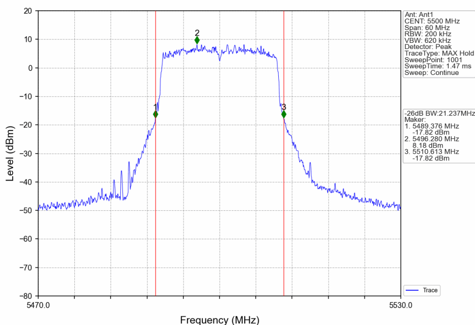
802.11ax(HEW20)_LCH_5500MHz_RU242_Left_Ant1_NTNV
