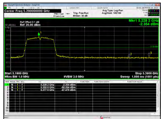
802.11n HT40
