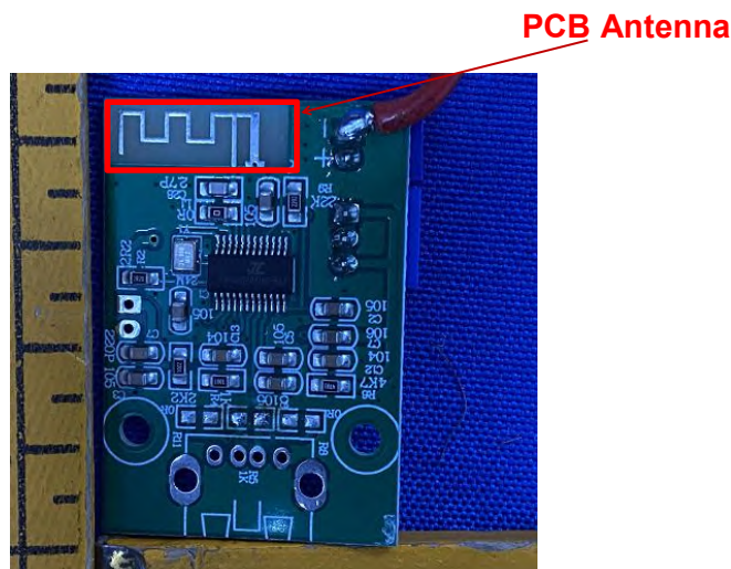
BDR+EDR Module
