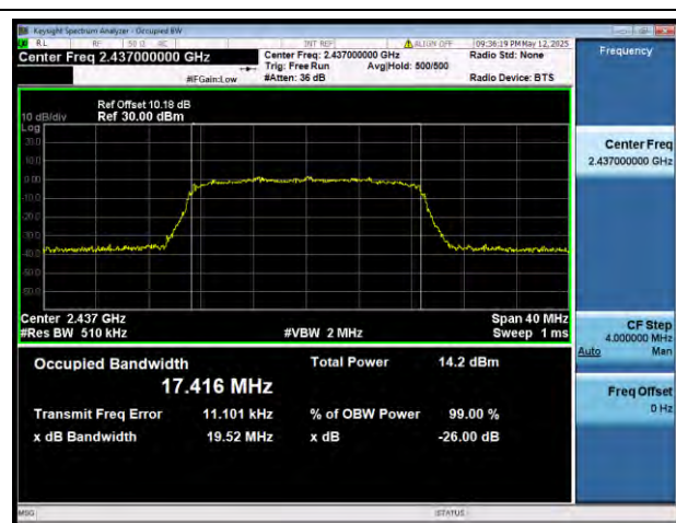
802.11g 6Mbps 2437MHz
