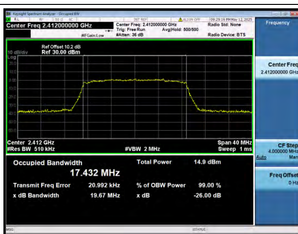
802.11g 6Mbps 2412MHz
