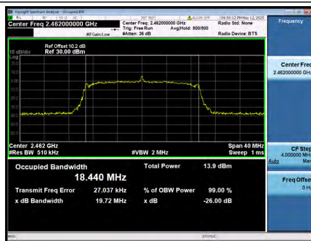
802.11n 6.5Mbps 2462MHz
