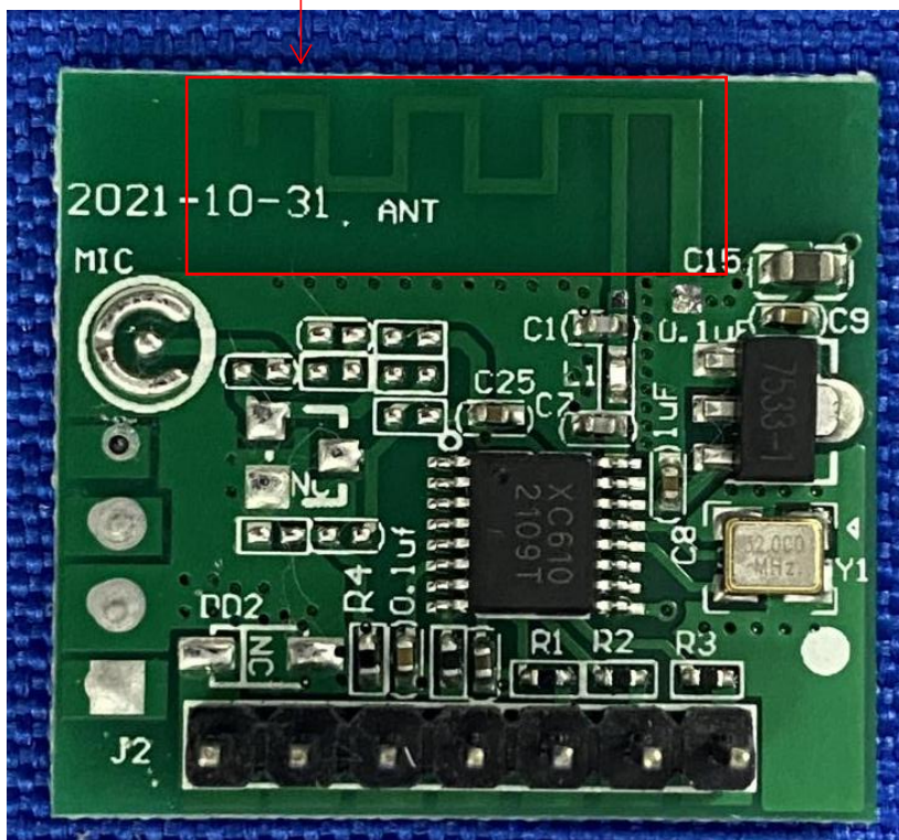
Antenna
