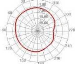
2400.000MHz E2
