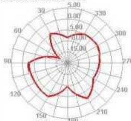
2450.000MHz E1
