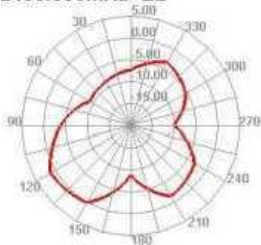
2400.000MHz E2
