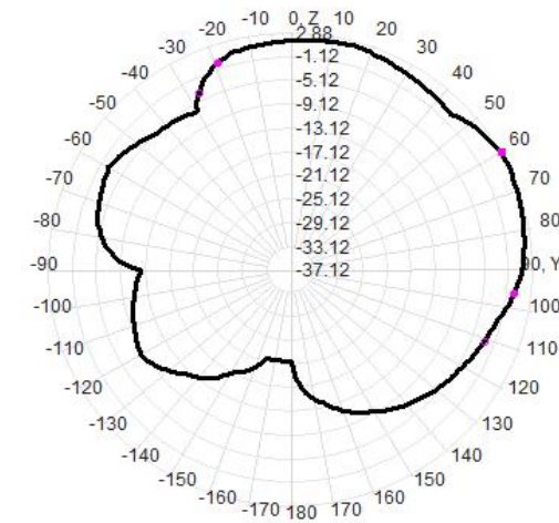
E2-YZ
