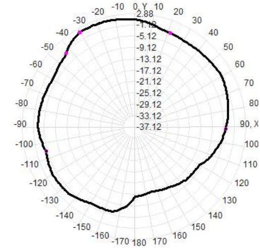
H-XY
