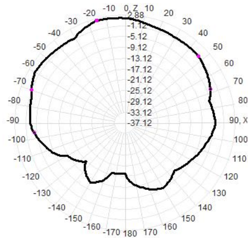
E1-XZ
