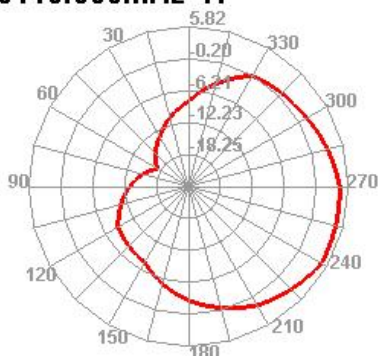
5110.000MHz H
