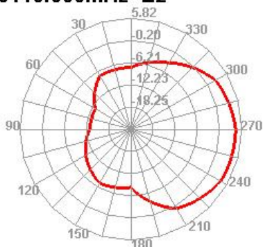
5110.000MHz E2
