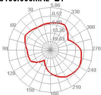
5100.000MHz E1
