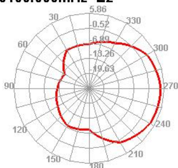
5100.000MHz E2
