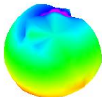
5100.000MHz E1
