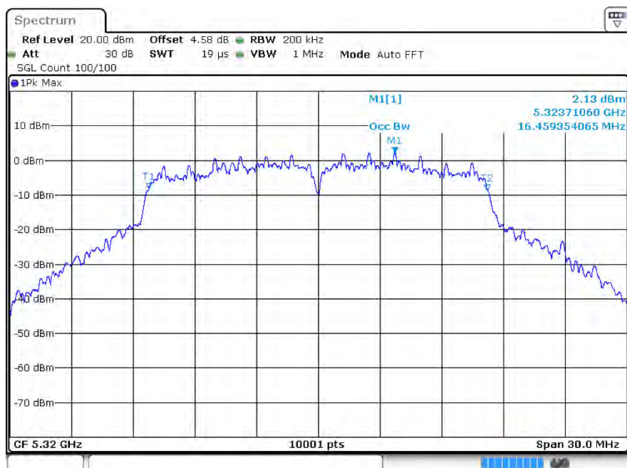
OBW a 5320MHz Ant1
