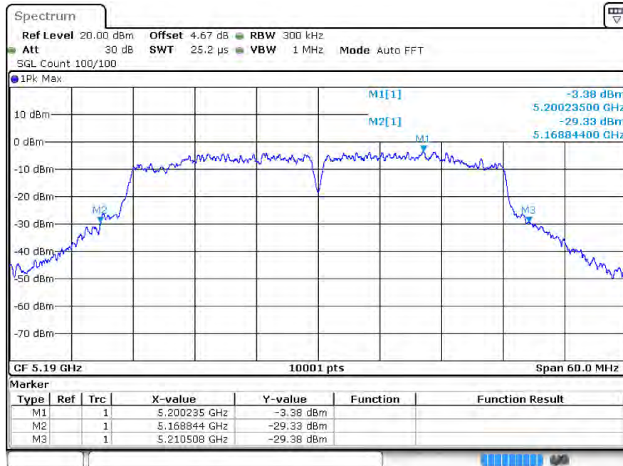
-26dB Bandwidthn40 5190MHz Ant1
