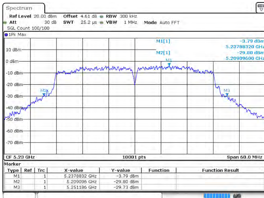
-26dB Bandwidthn40 5230MHz Ant1
