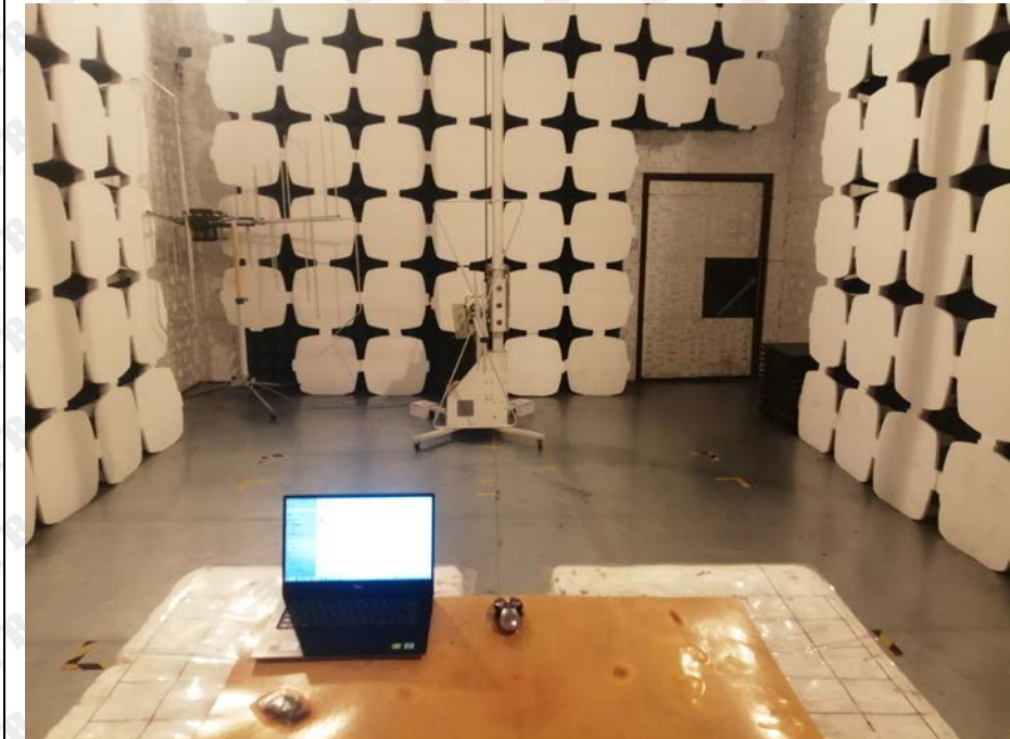
Below 1G
