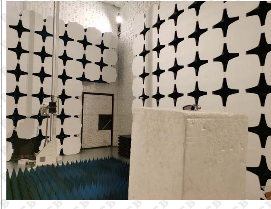
Above 1G
