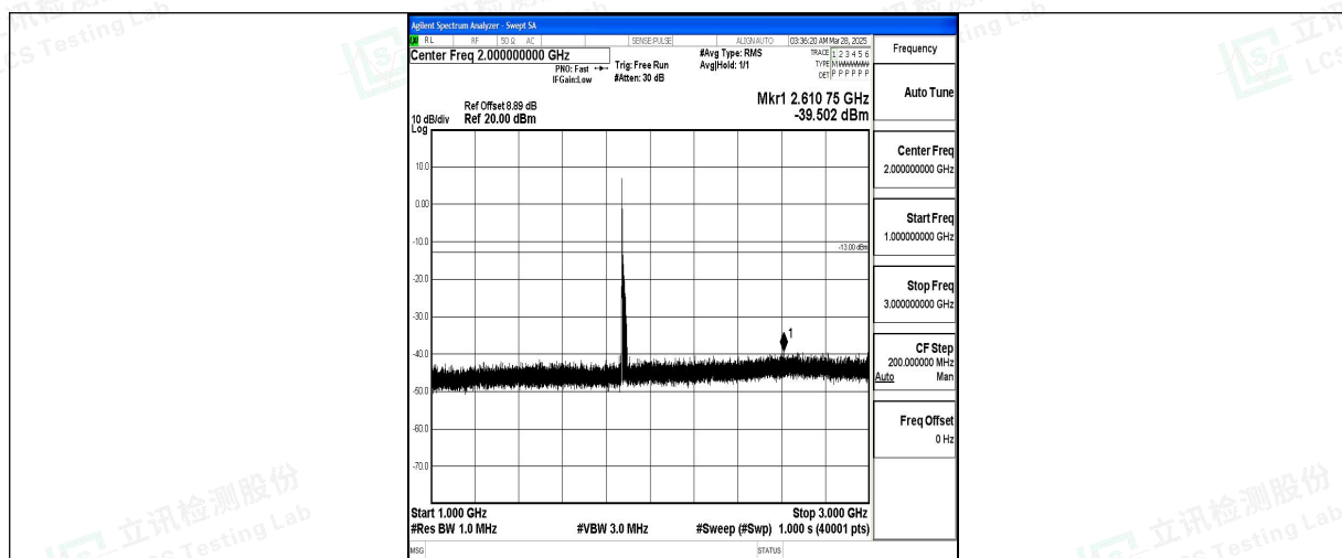
Band2 20MHz QPSK 18900 1RB#0 1000~3000 1000~3000
