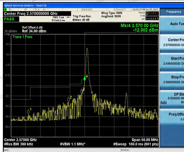
Band38-15MHz-QPSK-37825-1RB#74
