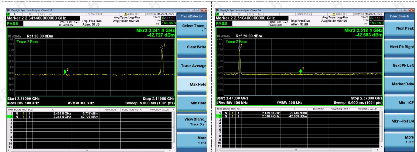
Left Band edge hopping off
