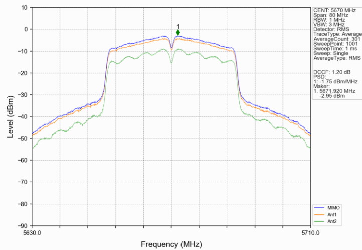
802.11n(HT40)_HCH_5670MHz MIMO NTNV
