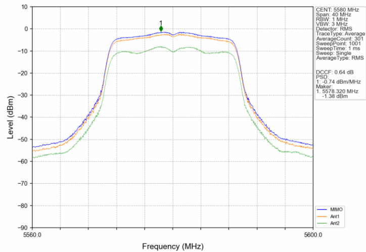
802.11n(HT20)_MCH_5580MHz MIMO NTN
