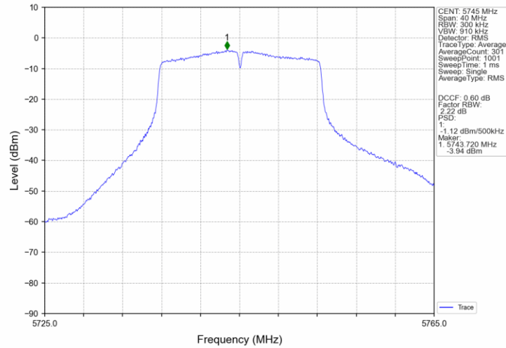
802.11a_LCH_5745MHz_Ant2_NTNV
