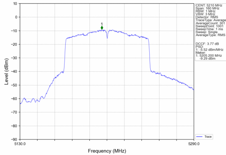
802.11ac(VHT80)_MCH_5210MHz_Ant2_NTNV
