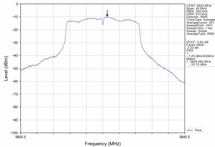
802.11n(HT20)_HCH_5825MHz_Ant2_NTNV
