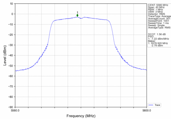
802.11ac(VHT20) MCH 5580MHz Ant1 NTN
