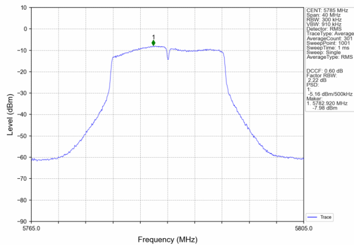
802.11a MCH 5785MHz Ant2 NTNv
