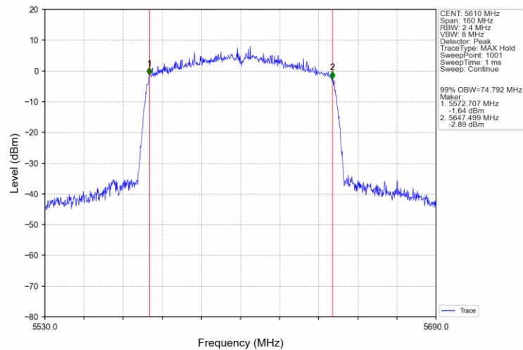
802.11ac(VHT80)_HCH_5610MHz_Ant0_NTNV
