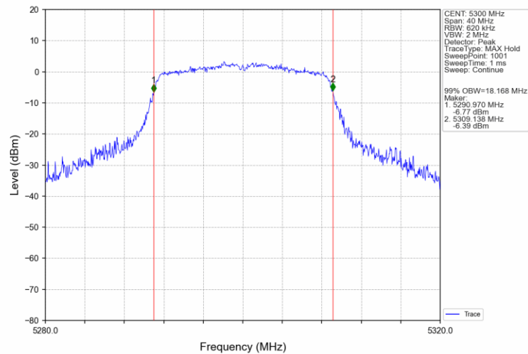
802.11ac(VHT20)_MCH_5300MHz_Ant0_NTNV
