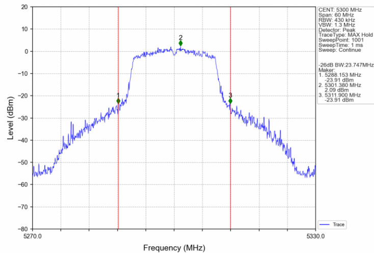
802.11n(HT20)_MCH_5300MHz_Ant0_NTNV
