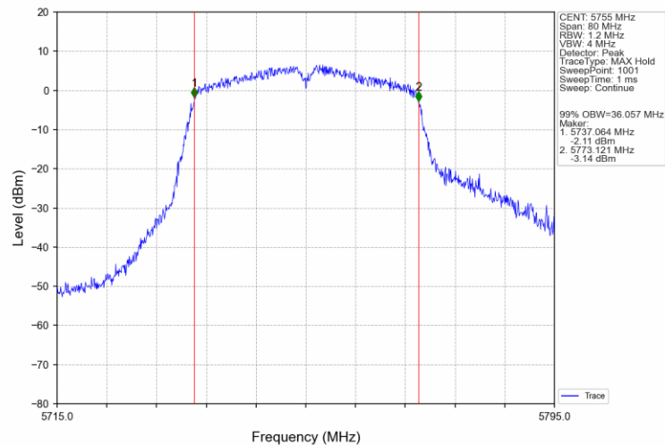
802.11n(HT40)_LCH_5755MHz_Ant0_NTNV
