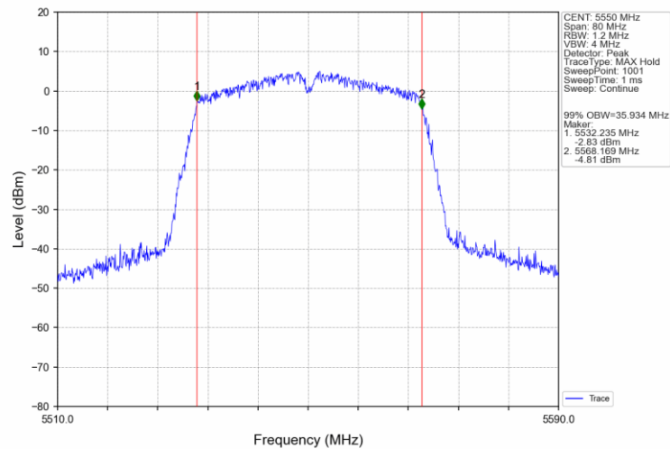
802.11n(HT40)_MCH_5550MHz_Ant0_NTNV
