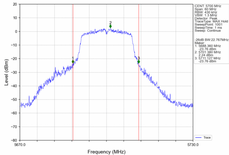
802.11n(HT20)_HCH_5700MHz_Ant0_NTNV
