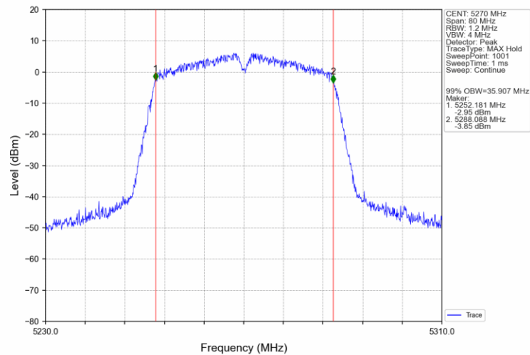
802.11ac(VHT40)_LCH_5270MHz_Ant0_NTNV
