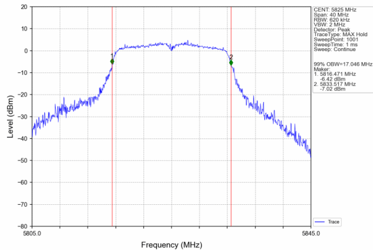
802.11a_HCH_5825MHz_Ant0_NTNV
