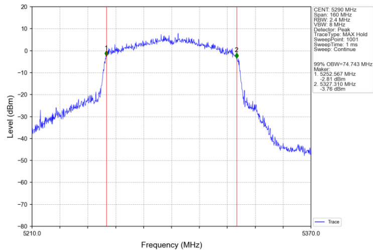
802.11ac(VHT80)_MCH_5290MHz_Ant0_NTNV
