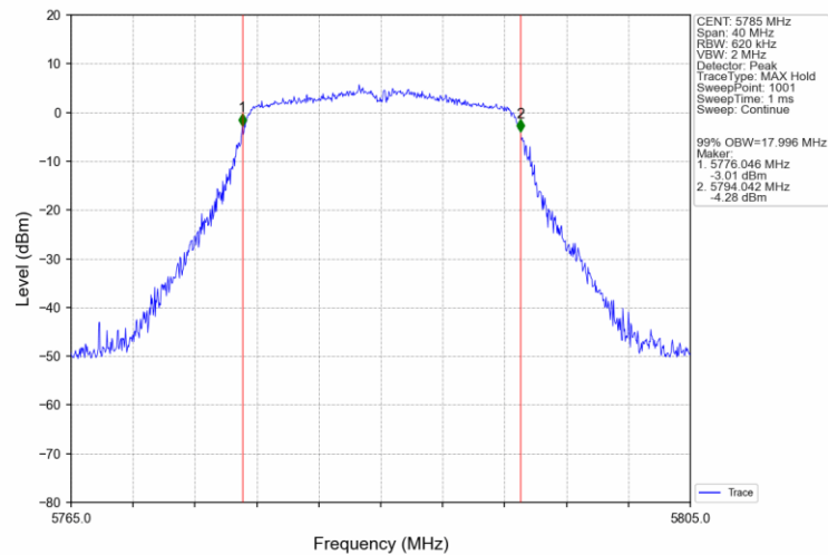
802.11ac(VHT20)_MCH_5785MHz_Ant0_NTNV
