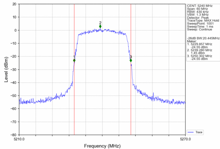
802.11n(HT20)_HCH_5240MHz_Ant0_NTNV
