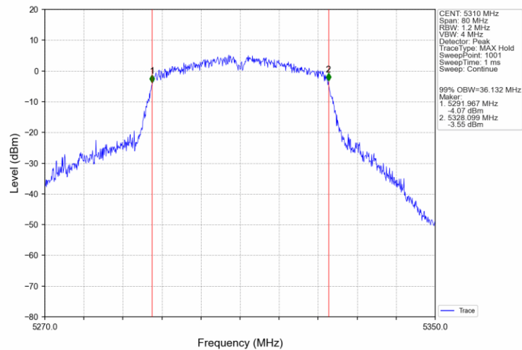
802.11n(HT40)_HCH_5310MHz_Ant0_NTNV
