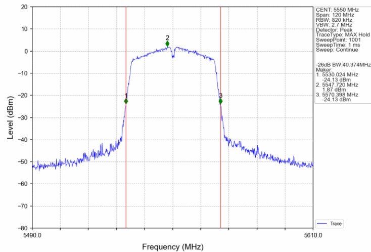
802.11n(HT40)_MCH_5550MHz_Ant0_NTNV
