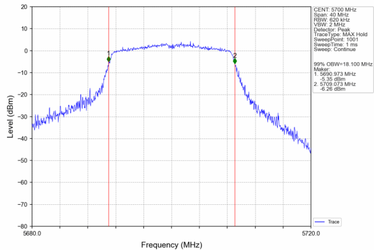
802.11ac(VHT20)_HCH_5700MHz_Ant0_NTNV
