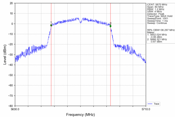
802.11ac(VHT40)_HCH_5670MHz_Ant0_NTNV
