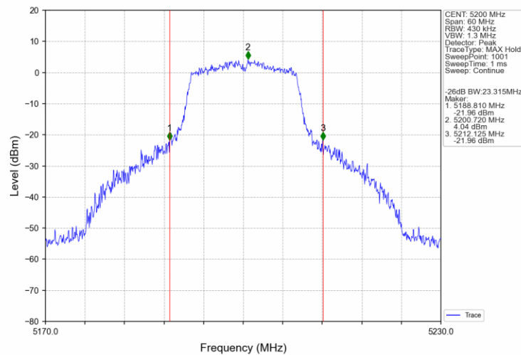
802.11a_MCH_5200MHz_Ant0_NTNV
