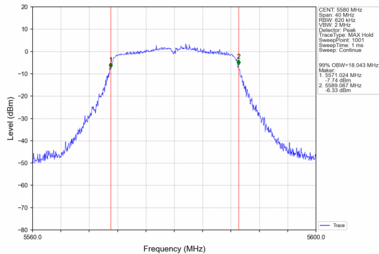
802.11n(HT20)_MCH_5580MHz_Ant0_NTNV
