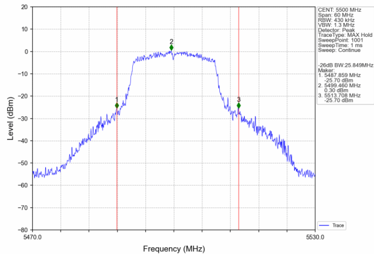
802.11n(HT20)_LCH_5500MHz_Ant0_NTNV
