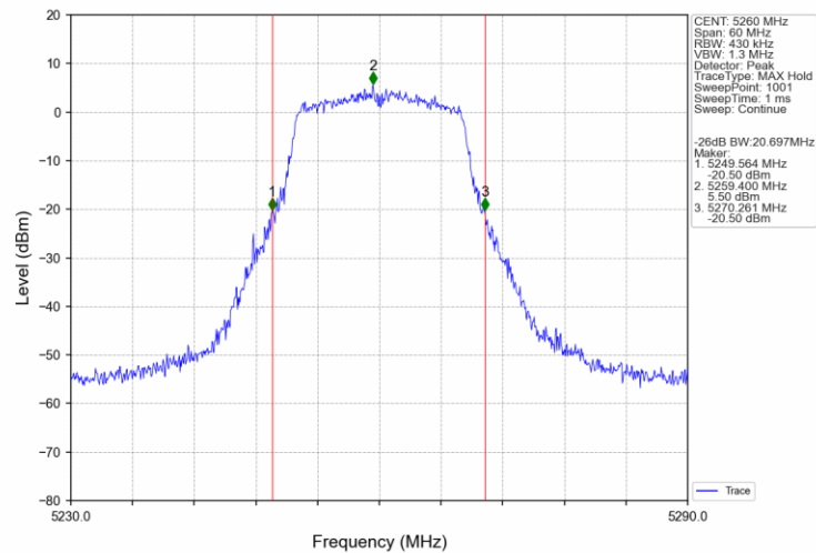
802.11a_LCH_5260MHz_Ant0_NTNV
