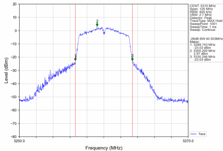
802.11n(HT40)_HCH_5310MHz_Ant0_NTNV
