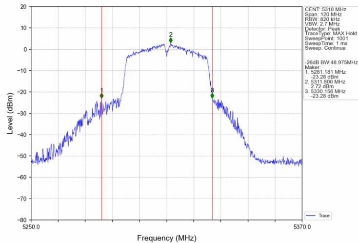
802.11ac(VHT40)_HCH_5310MHz_Ant0_NTNV
