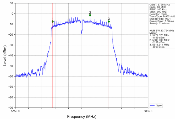
802.11n(HT40)_HCH_5795MHz_Ant0_NTNV
