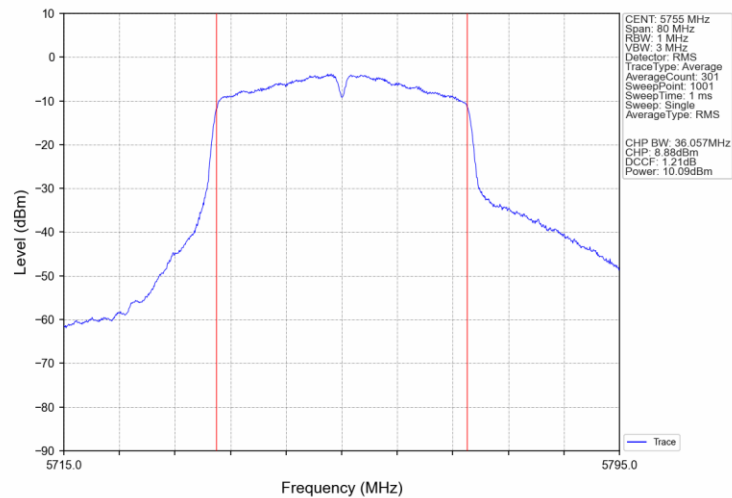
802.11n(HT40)_LCH_5755MHz_Ant0_NTNV
