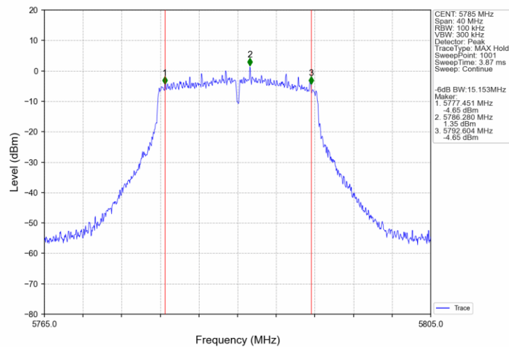
802.11a_MCH_5785MHz_Ant0_NTNV
