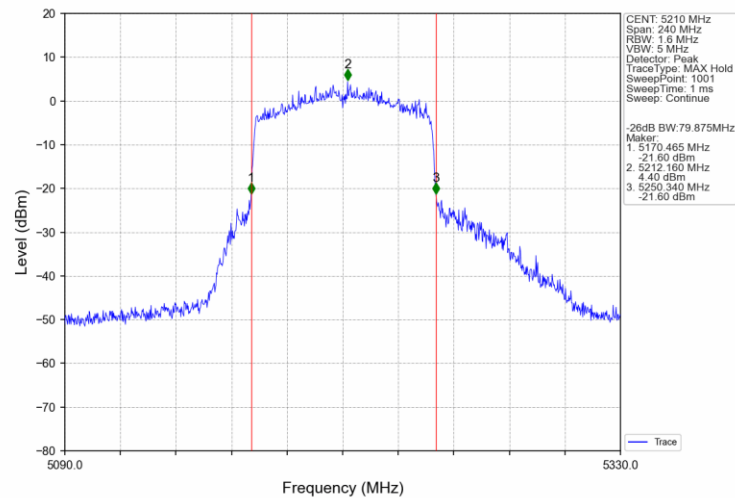
802.11ac(VHT80)_MCH_5210MHz_Ant0_NTNV
