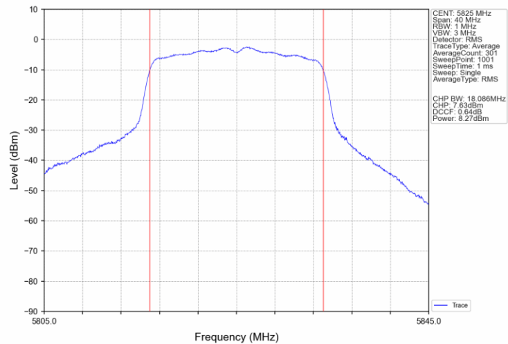
802.11n(HT20)_HCH_5825MHz_Ant0_NTNV
