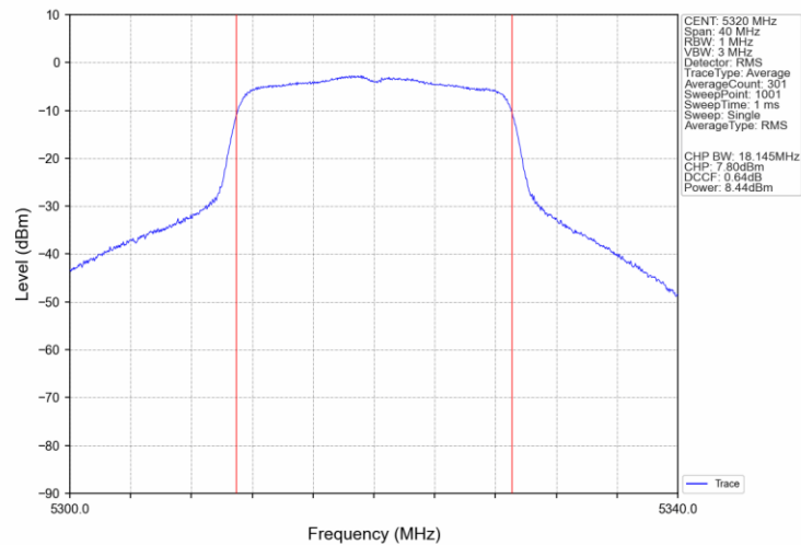
802.11n(HT20)_HCH_5320MHz_Ant0_NTNV
