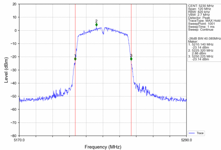
802.11ac(VHT40)_HCH_5230MHz_Ant0_NTNV
