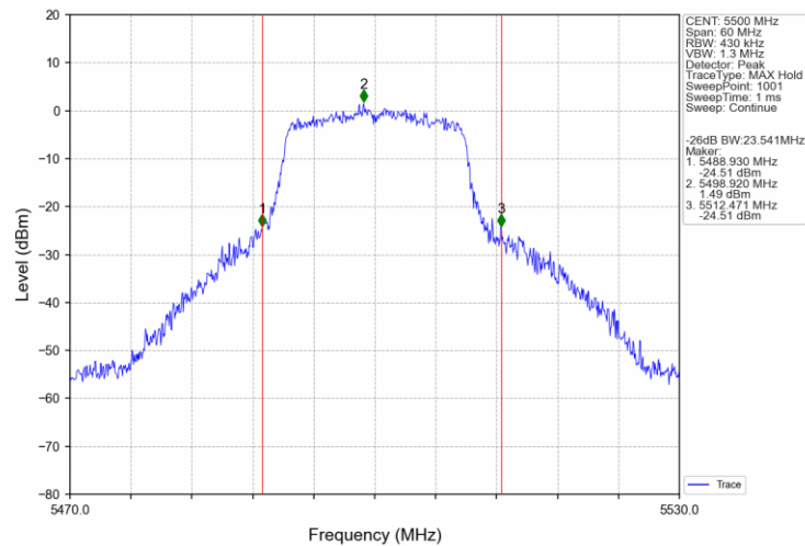
802.11ac(VHT20)_LCH_5500MHz_Ant0_NTNV
