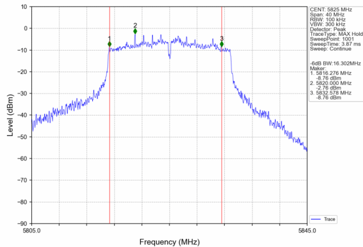
802.11n(HT20)_HCH_5825MHz_Ant0_NTNV
