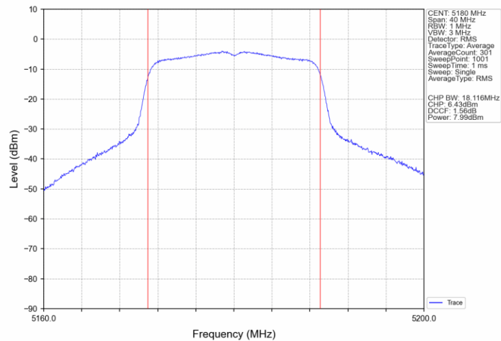
802.11ac(VHT20)_LCH_5180MHz_Ant0_NTNV
