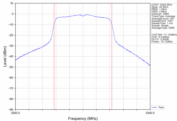
802.11a_HCH_5320MHz_Ant0_NTNV
