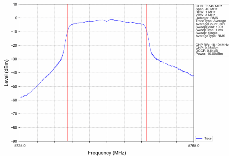
802.11n(HT20)_LCH_5745MHz_Ant0_NTNV
