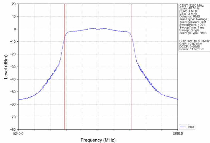
802.11a_LCH_5260MHz_Ant0_NTNV
