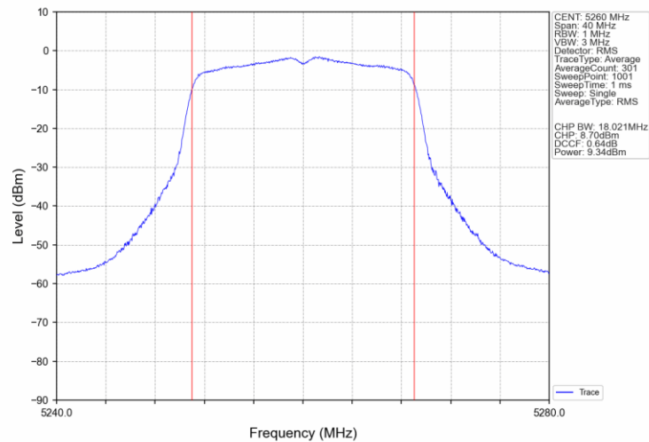
802.11n(HT20)_LCH_5260MHz_Ant0_NTNV
