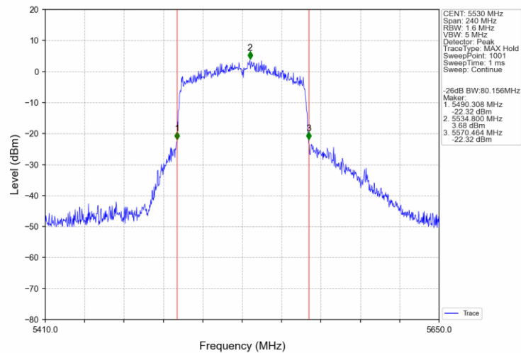
802.11ac(VHT80)_LCH_5530MHz_Ant0_NTNV
