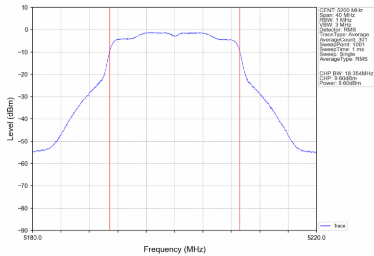
802.11n(HT20) MCH 5200MHz Ant1 NTN
