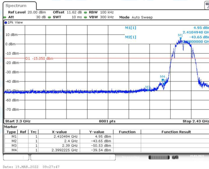
11B_Ant1_Low_2412
