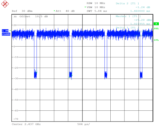
g_2437MHz_Chain 0 1.366 ms,1.46ms
